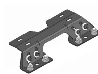
KIT DE FIXATIONS UNIVERSELLES POUR RAMPE FX - PAR PERÇAGE DU TOIT
