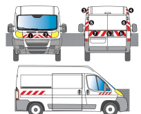
KIT R-B CL. A AVT+ARR+LAT - CITROËN JUMPER H2 TÔLÉ (2006-2013)
