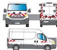
KIT ROUGE BLANC CL. A STANDARD - IVECO DAILY H2 (2014-2023)
