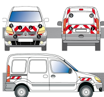
KIT R-B CL. A AVT+ARR+LAT - RENAULT KANGOO À HAYON (2003-2007)
