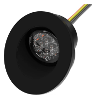
FEU DE PARE-BRISE BB4 - 4 LEDS - 60°
